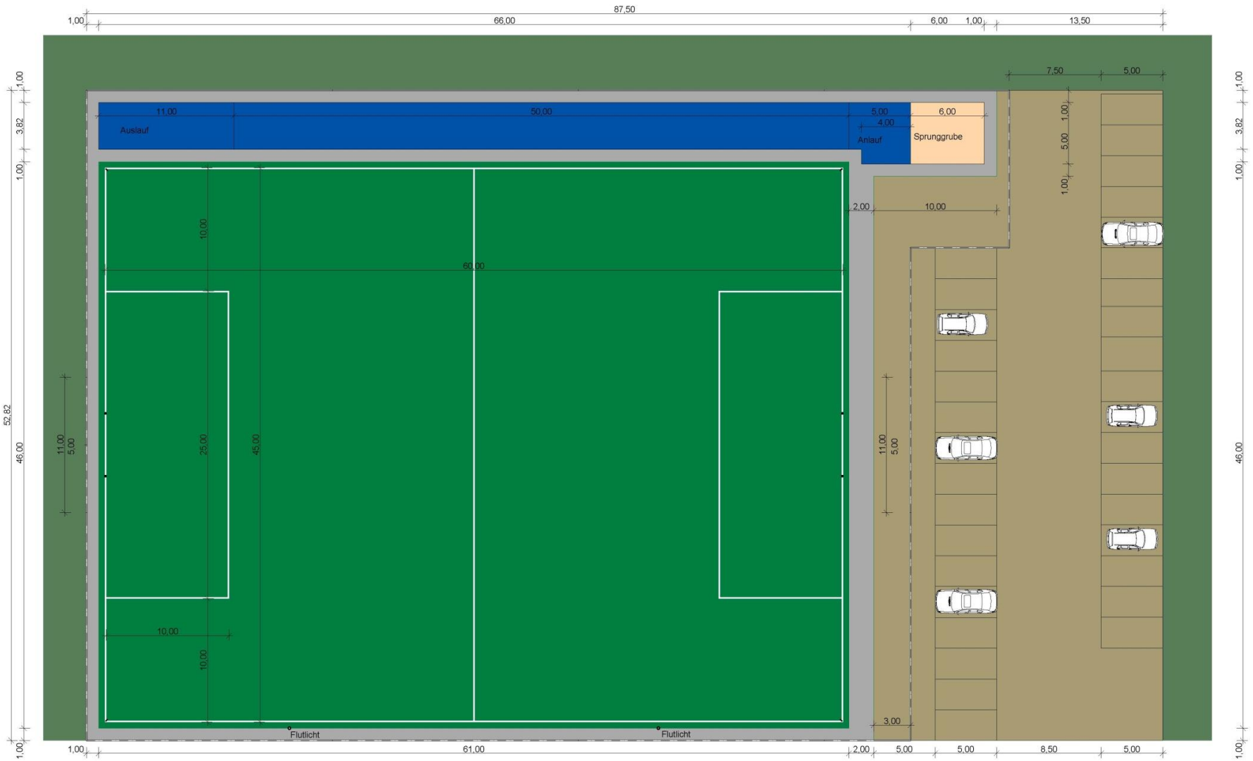
Umgestaltung des Sportplatzes Schwalmtal-Brauerschwend M.: 1/200
